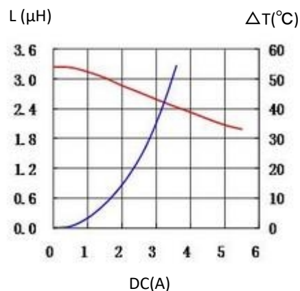
9. 0415CDMCCDS-3R3MC
