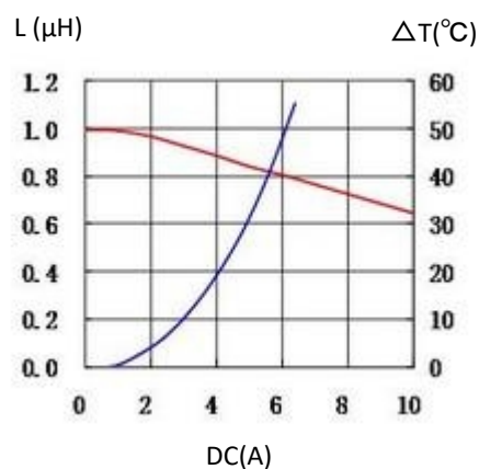
6. 0415CDMCCDS-1R0MC
