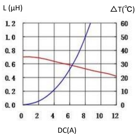
5. 0415CDMCCDS-R68MC
