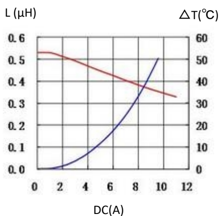
4. 0415CDMCCDS-R56MC
